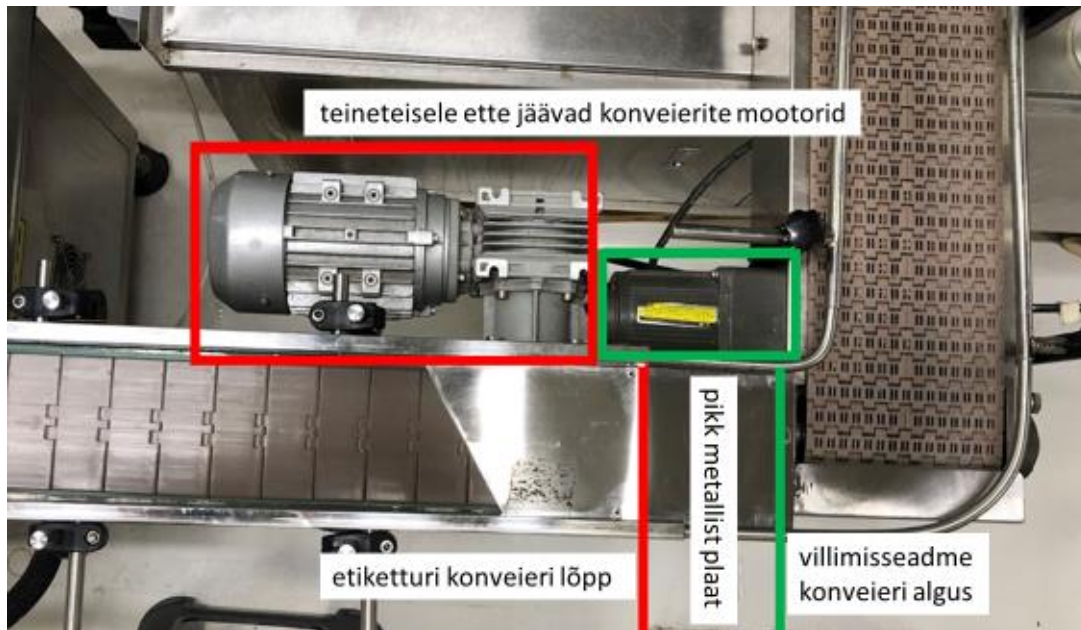
Joonis 3. Teineteisele ette jäävad konveierite mootorid
