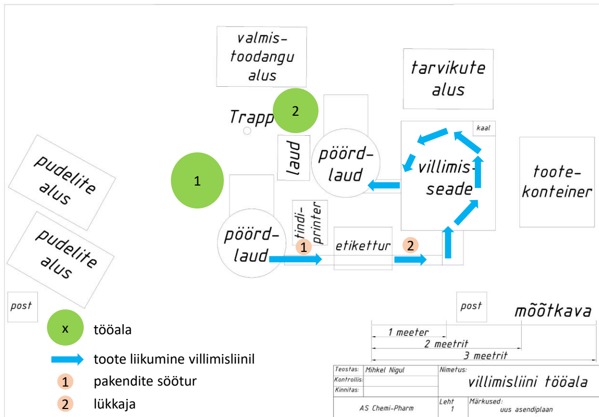
Joonis 4. Villimisliini uus asendiplaan
