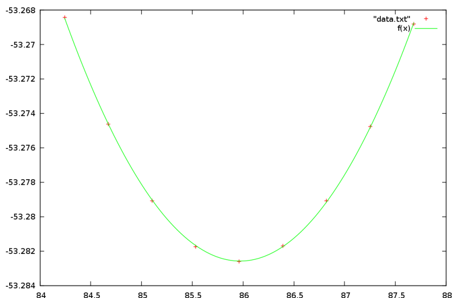
Joonis 2: Arvutuspunktid maatriksi D_2 jaoks, venitusel 2%
