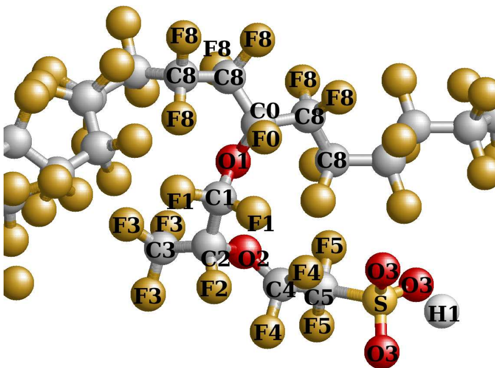
Joonis 1: Lõik Nafioni ® ahelast. Aatomid C8 ja F8 kuuluvad peeahelasse, ülejäänud kõrvalahelasse.
